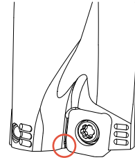
Abb. 7 Bruch der Wendeschneidplatte nahe dem Bohrerzentrum
